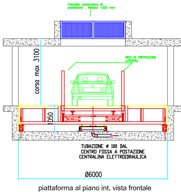
piattaforma al piano int. vista frontale
