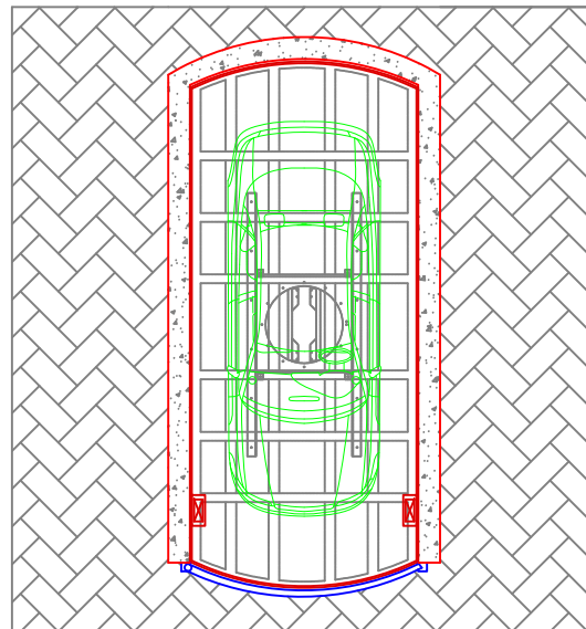
piattaforma al piano terra vista in pianta
