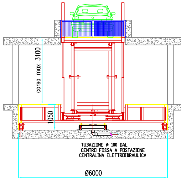
piattaforma al piano terra vista frontale
