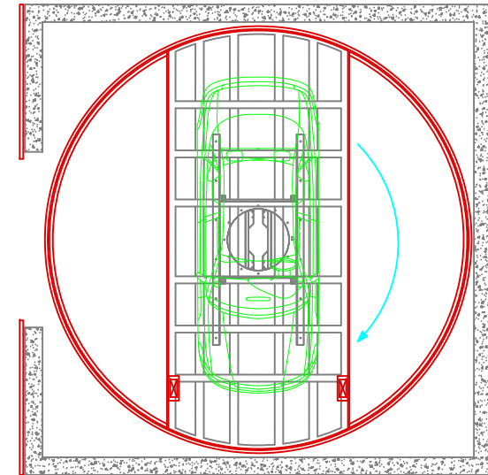
piattaforma al piano int. in posizione di salita
