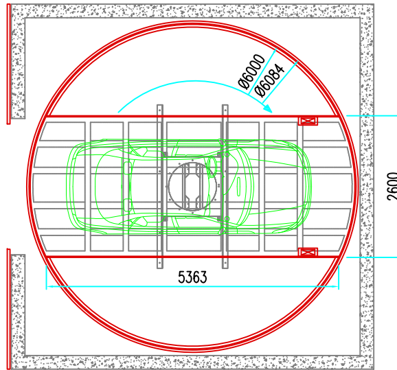
piattaforma al piano int. vista in pianta
