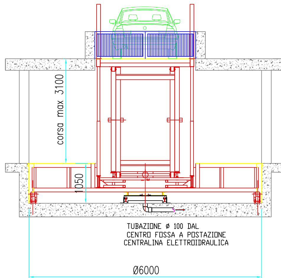
piattaforma al piano terra vista frontale
