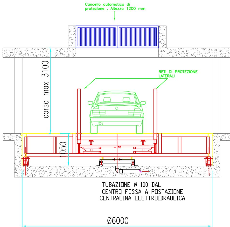
piattaforma al piano int. vista frontale
